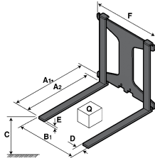
FA: säädettävät haarukat
